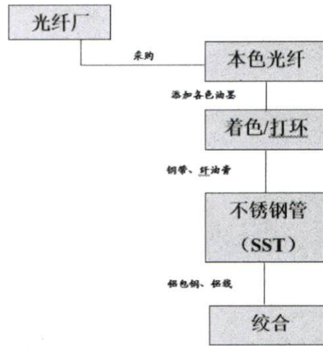
图 3-2 OPPC 工艺流程图
