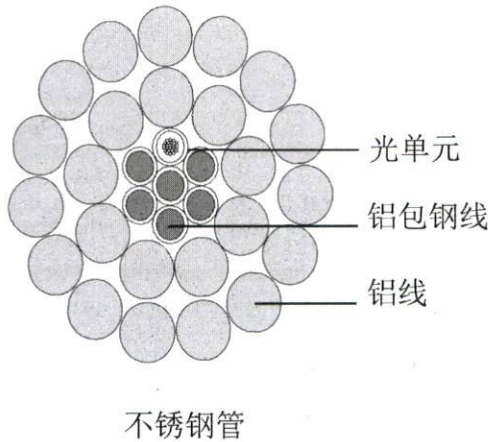
图 2 OPPC 光纤复合架空相线
